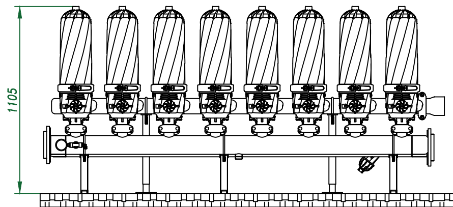
Вид спереди
