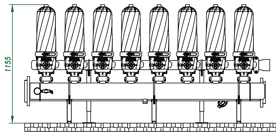
Вид спереди
