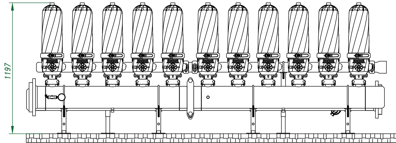
Вид спереди
