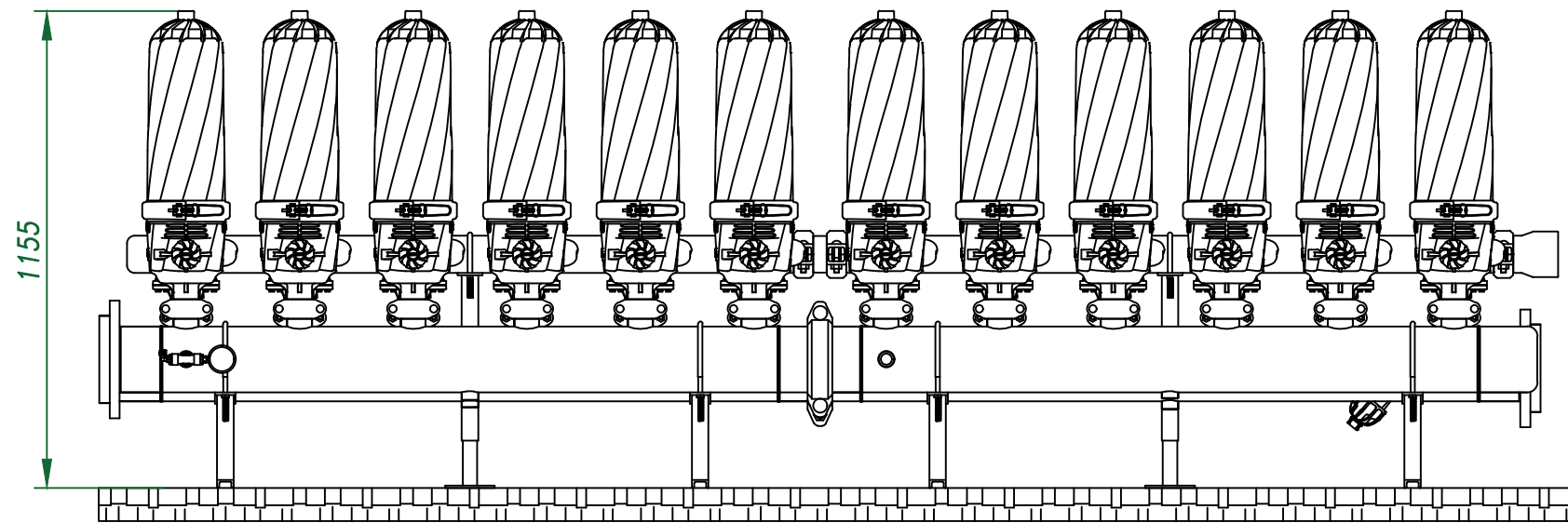
Вид спереди
